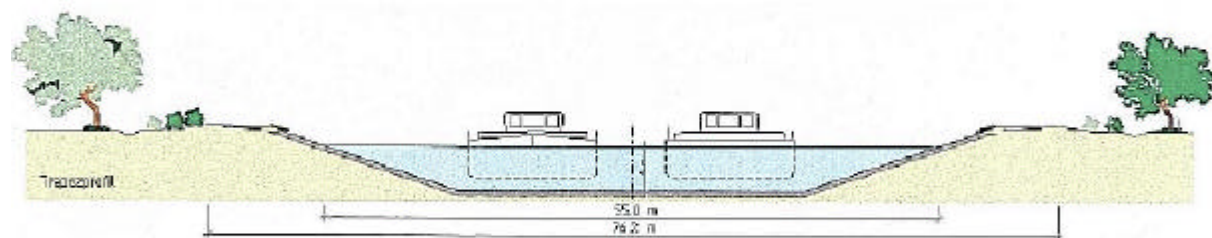
Trapezprofil
