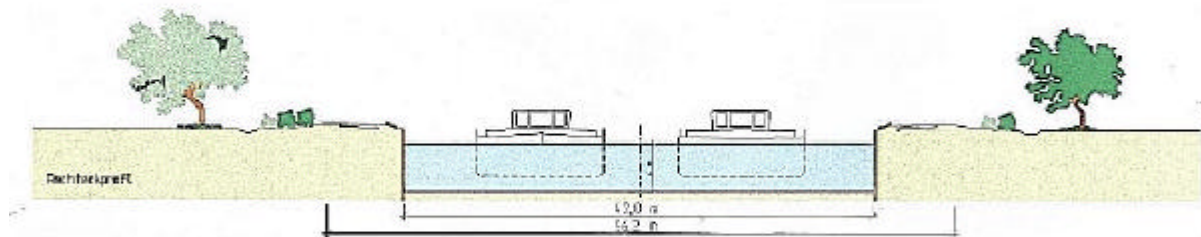
Rechteck-Profil
