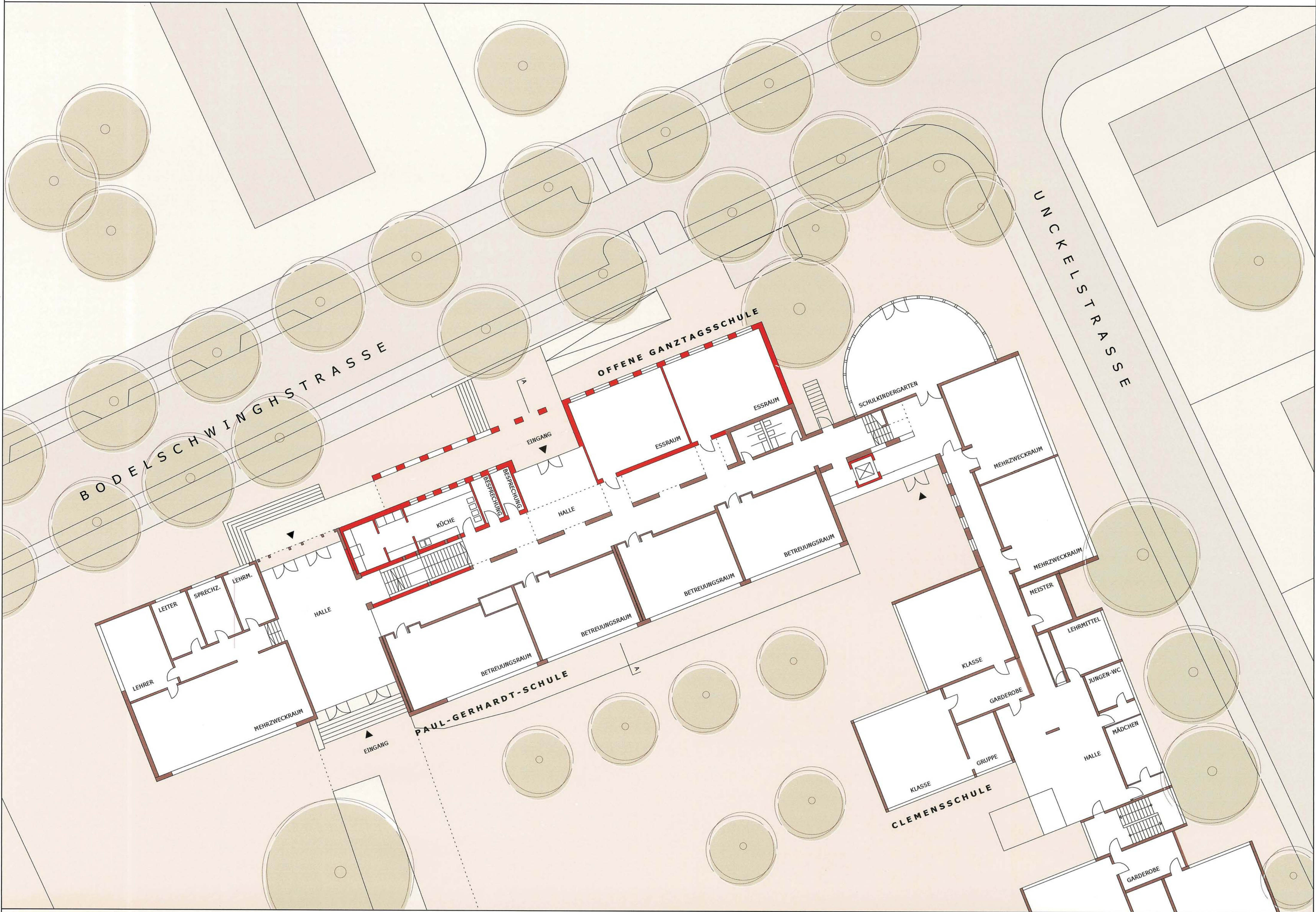
GRUNDRISS EG M.1:200
