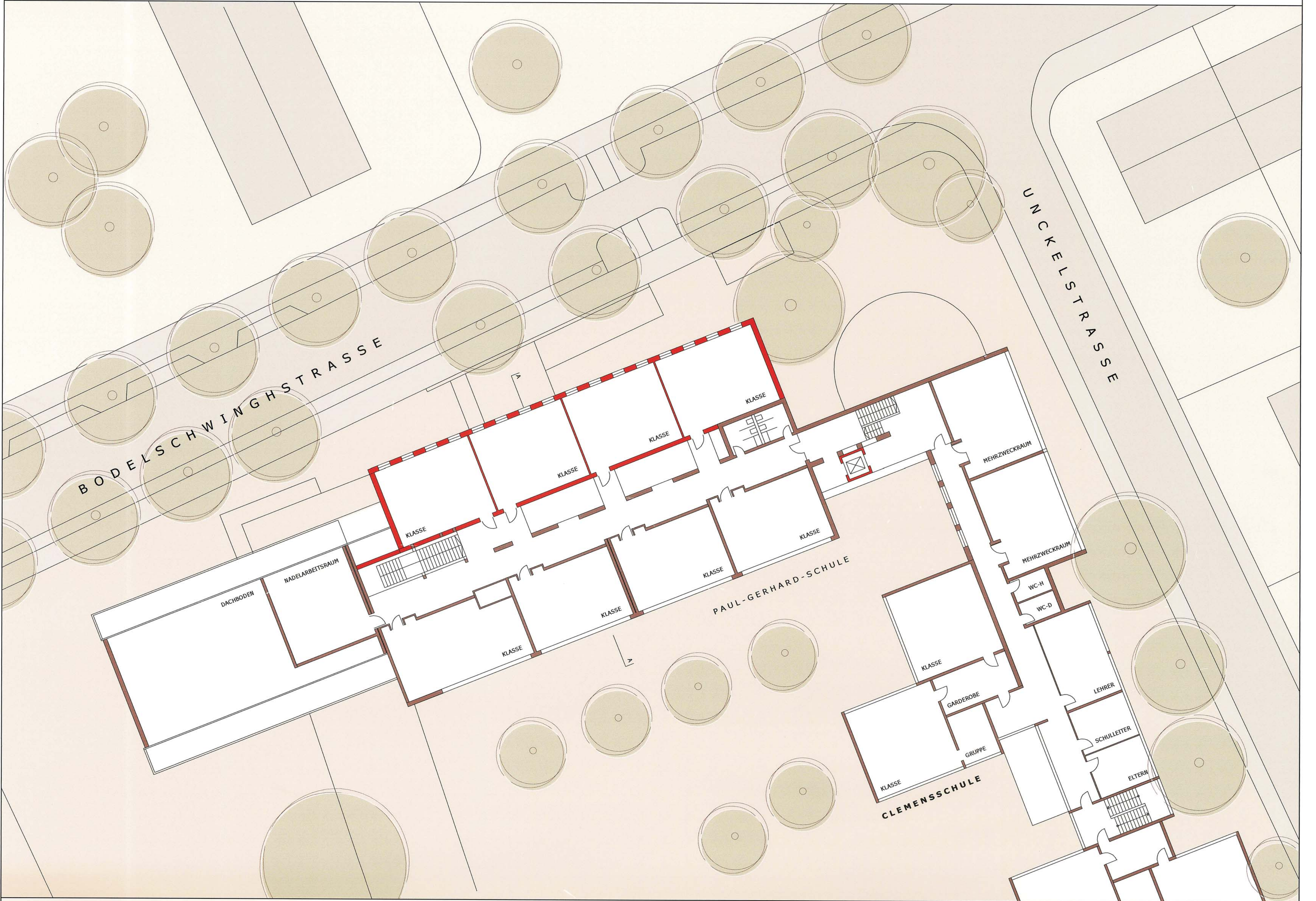
GRUNDRISS OG M.1:200
