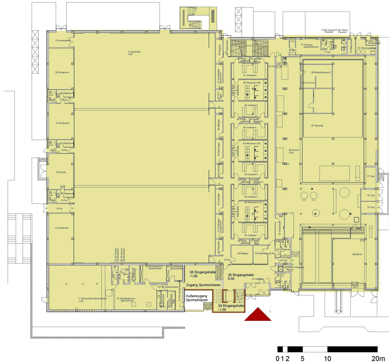
G06070 Bäderkonzept Münster Hallenbad Hiltrup Erdgeschoss
