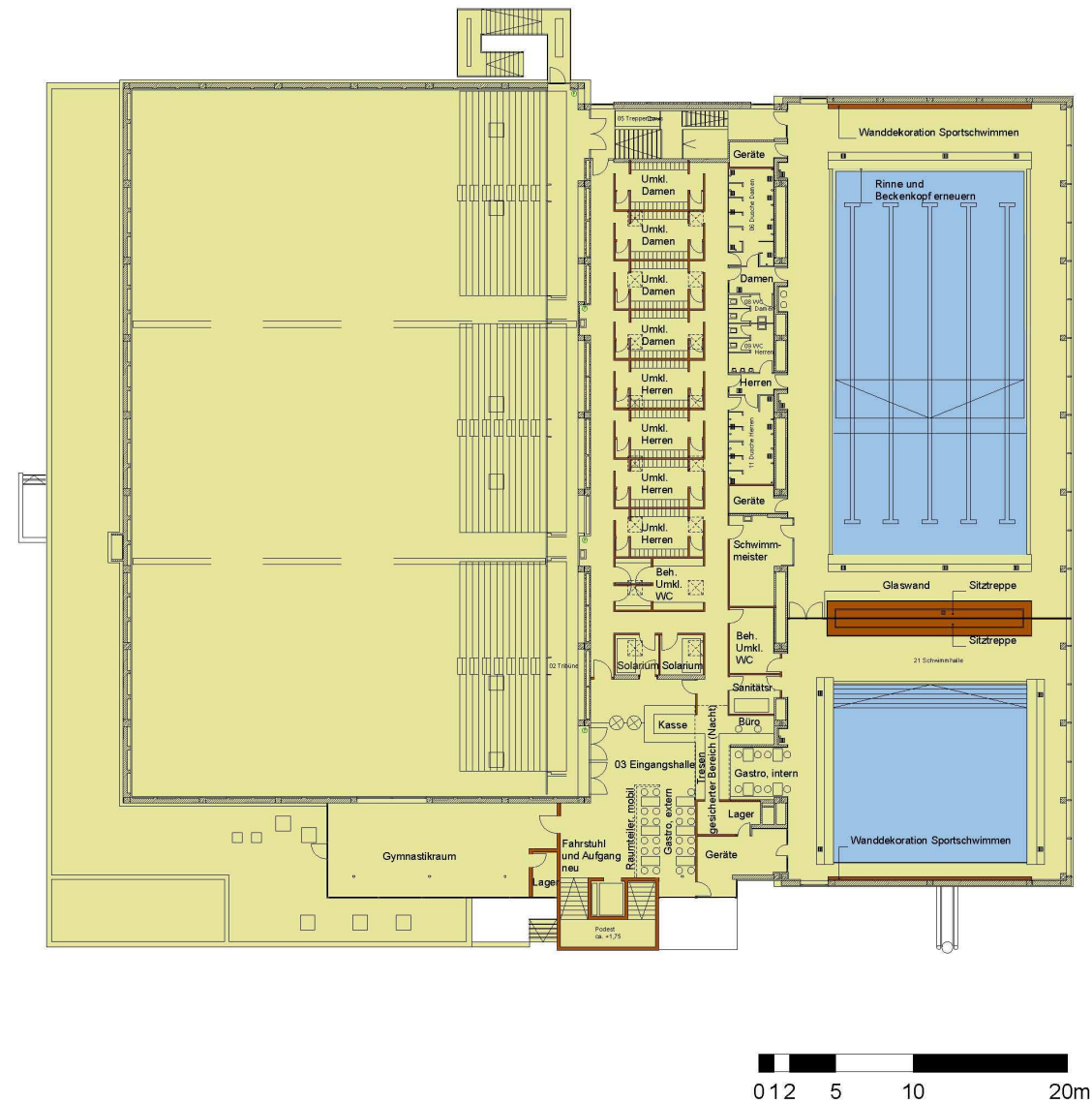
G06070 Bäderkonzept Münster Hallenbad Hiltrup Obergeschoss
