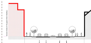
Querschnitt B – B Höhe Bio-Supermarkt
