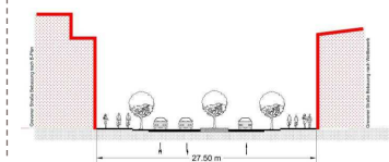
Querschnitt D – D Höhe Nr. 31 / Neubau
