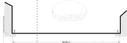
Querschnitt B – B Höhe Bio-Supermarkt
