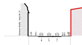
Querschnitt D – D Höhe Nr. 31 / Erhalt
