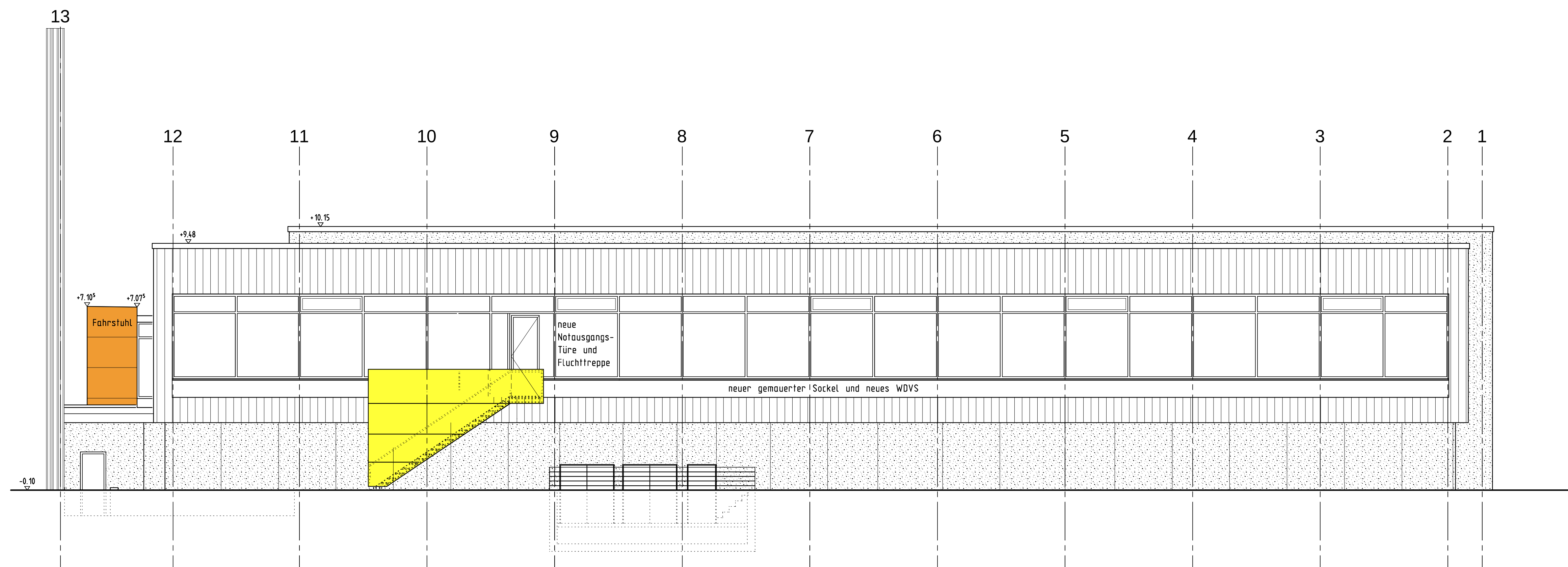
Westansicht
