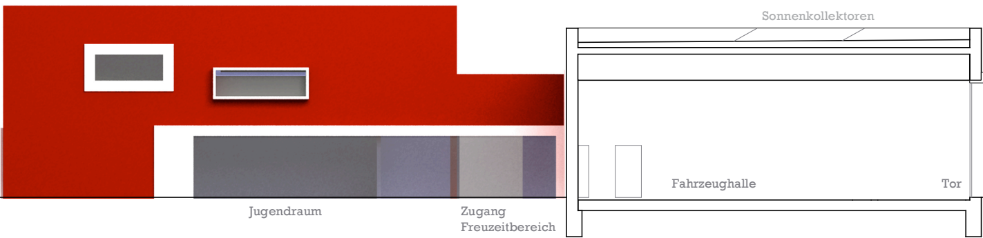
schnitt dd
