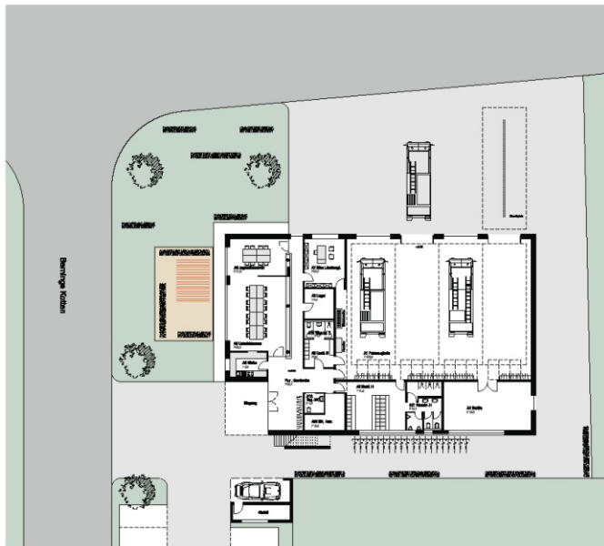
Grundriss Erdgeschoss
