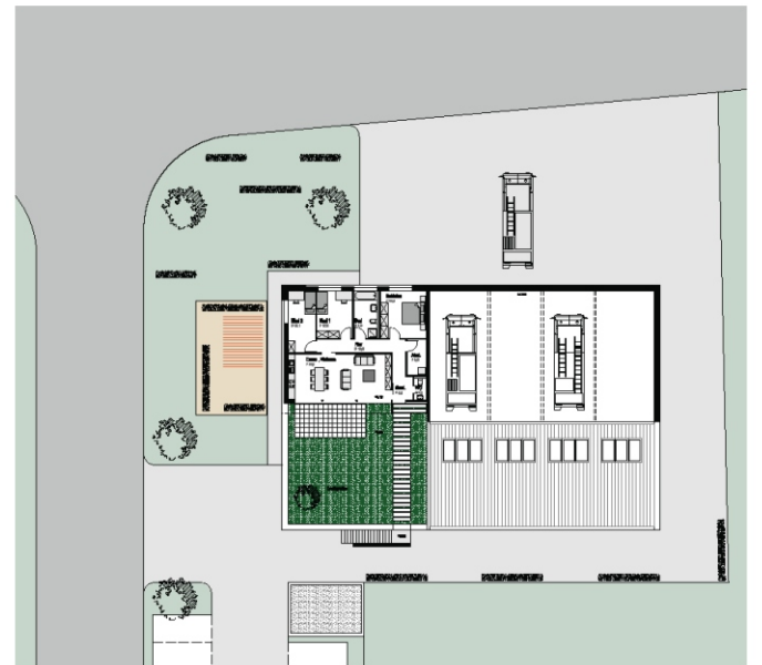
Grundriss Dachgeschoss
