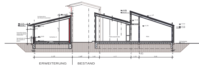
SCHNITT B-B
