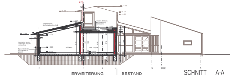
SCHNITT A-A
