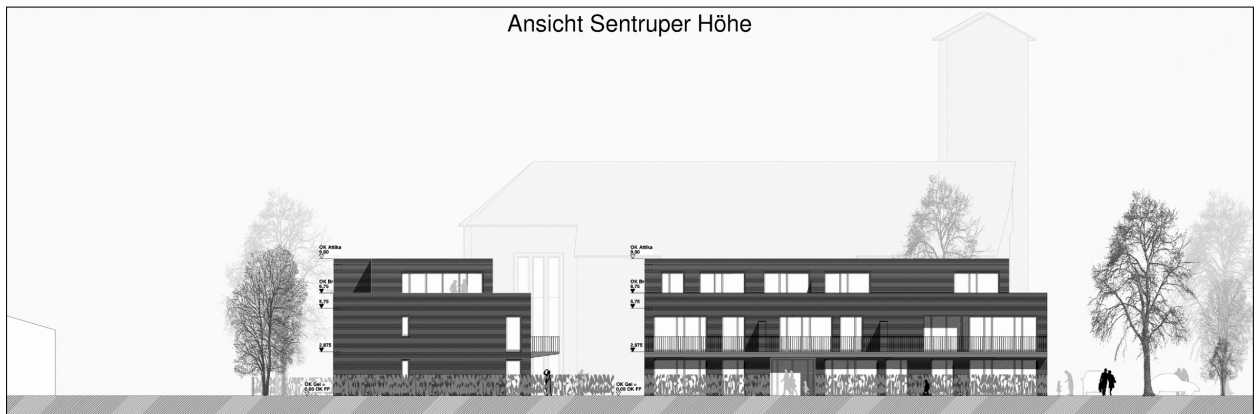
Ansicht Nordwest
