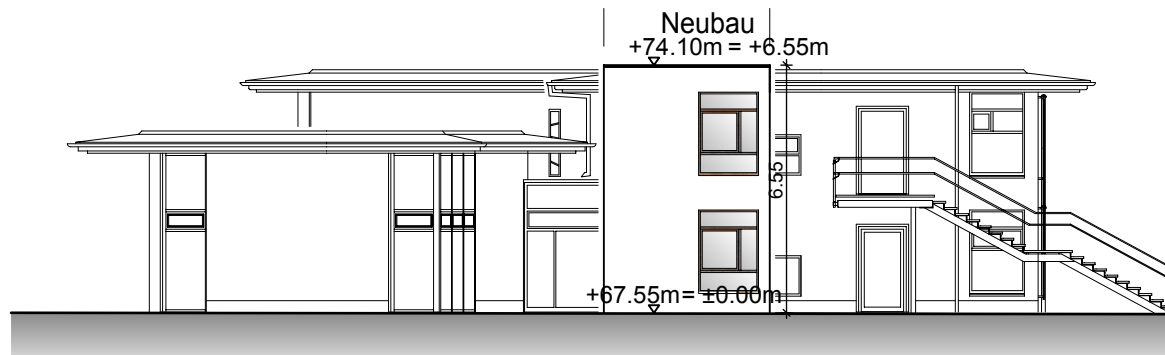
OST Ansicht
