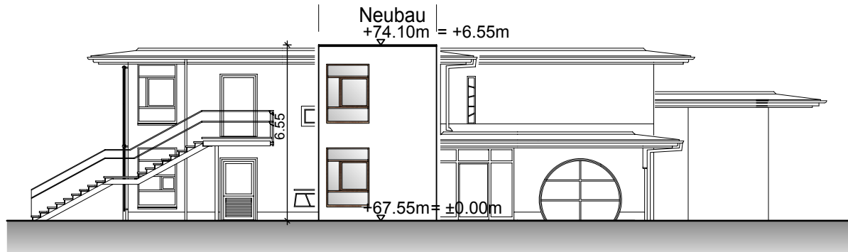
WEST Ansicht
