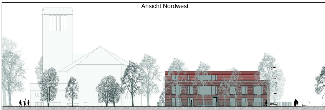
Ansicht / Schnitt Nordost
