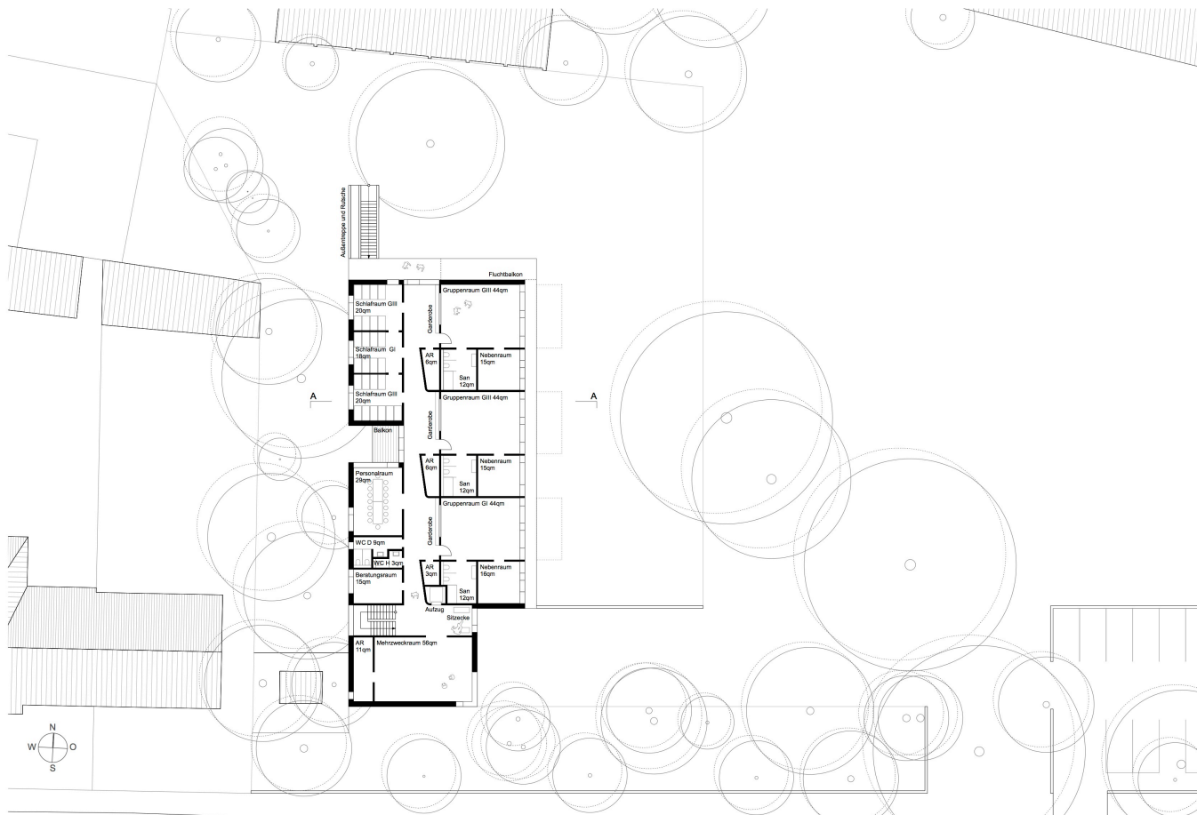
Obergeschoss // M 1:200
