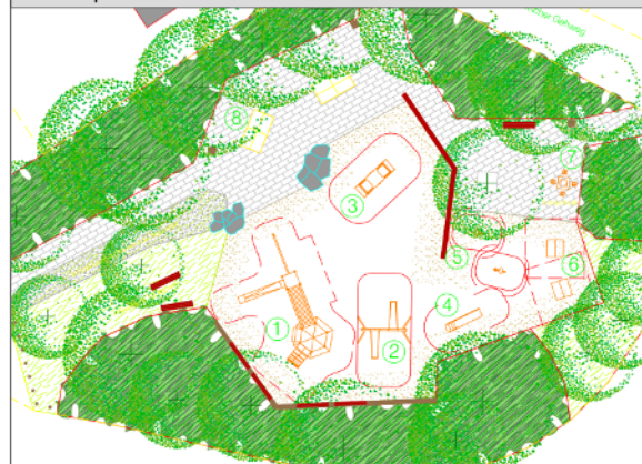
Bestandsplan M 1:200
