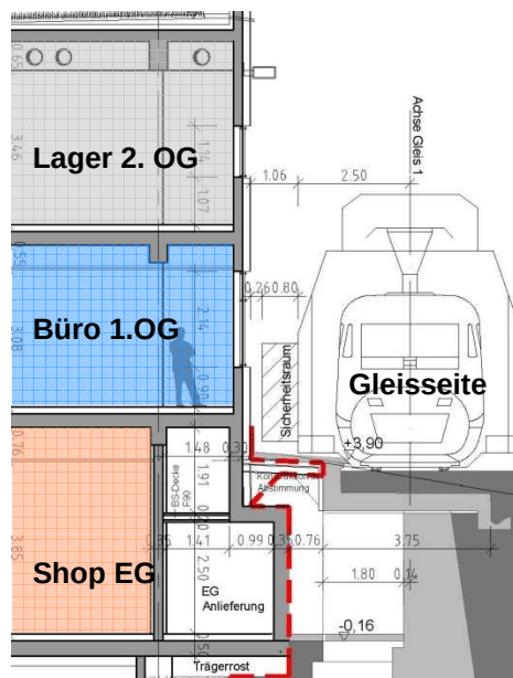
Fassadeschnitt
