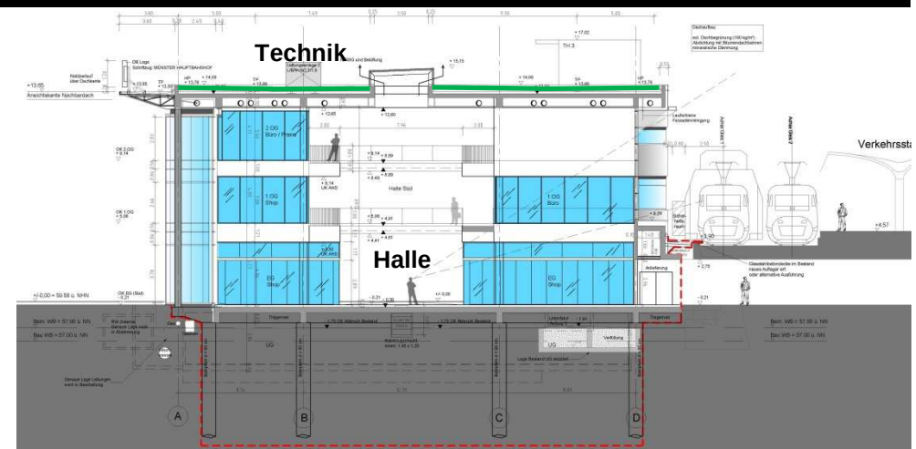
Schnitt B-B
