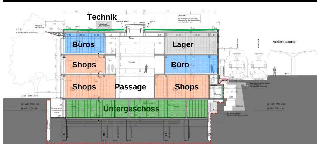
Schnitt A-A
