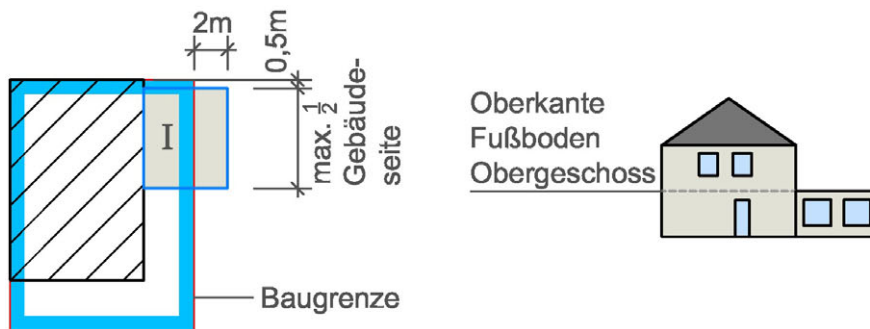
Abbildung 8: Mögliche Überschreitung der Baugrenzen (Beispiel)
