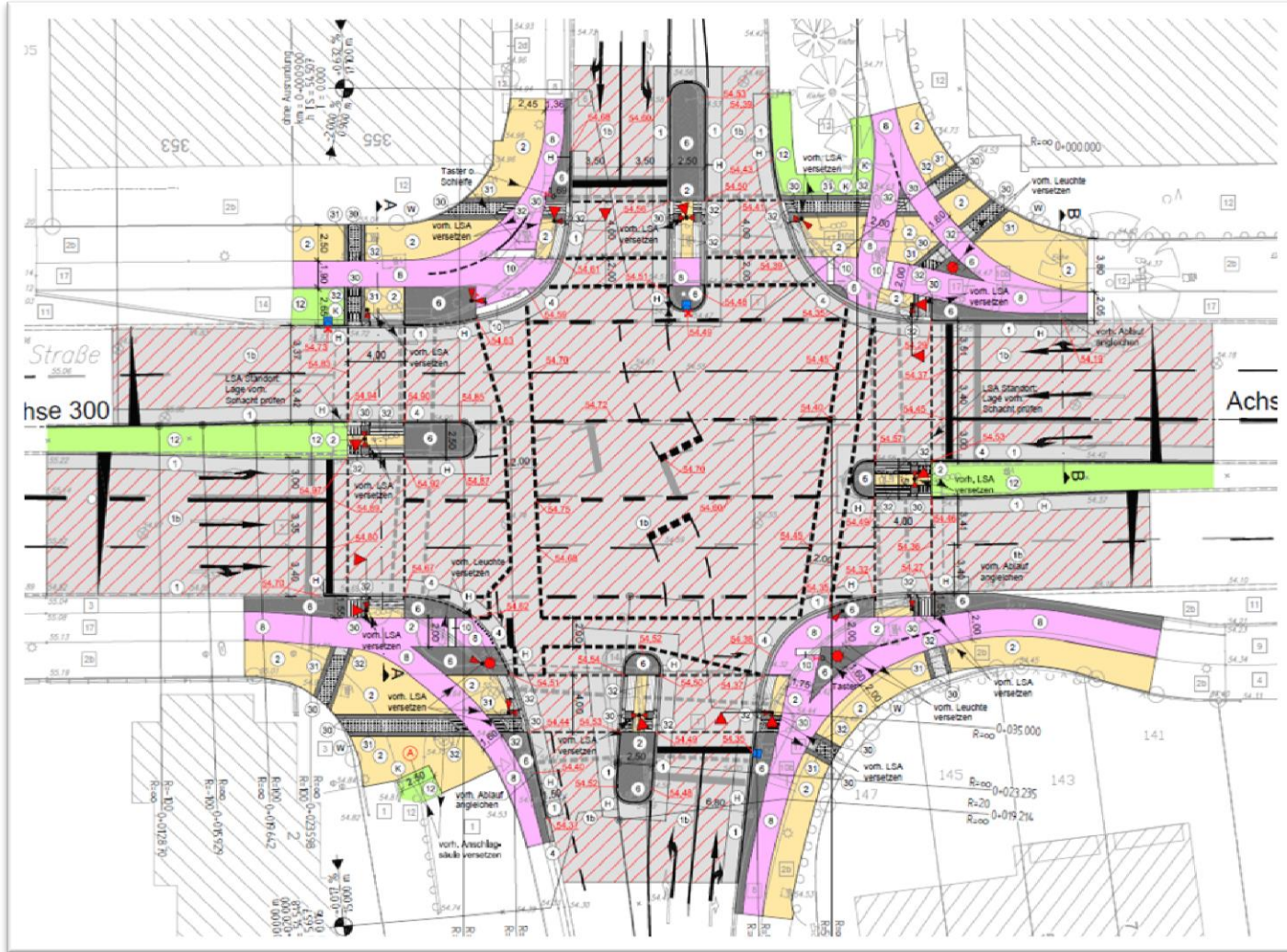
Anlage zur Vorlage V/0997/2015: Greverer Straße – York-Ring bis Kanalstraße: Kreuzung Kristiansandstraße / Wangeroogweg - Baubeschluss Straßenbau
