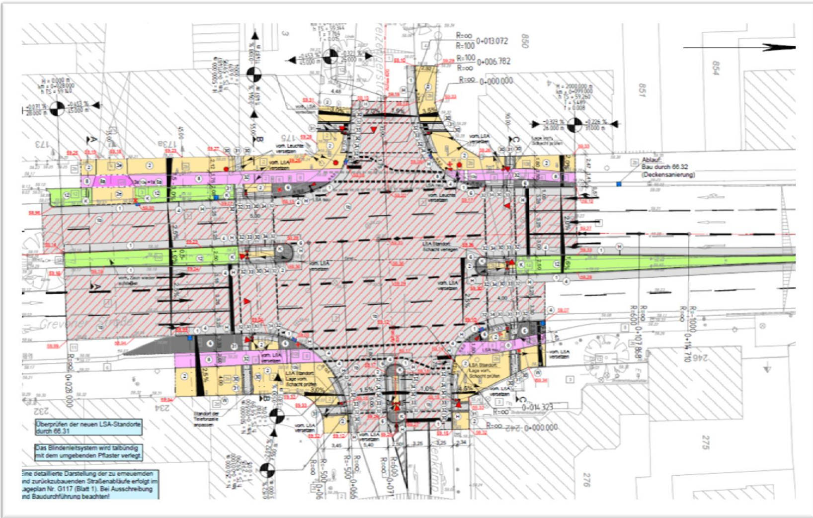
Anlage zur Vorlage V/1012/2015: Grevener Straße – York-Ring bis Kanalstraße: Kreuzung Dreizehnerstraße / Nienkamp - Baubeschluss Straßenbau
