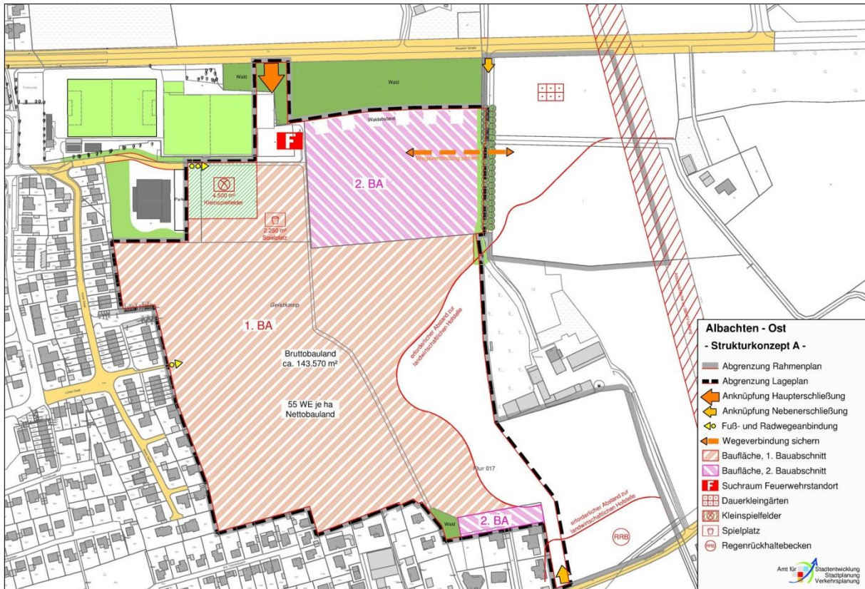
Strukturkonzept A:
