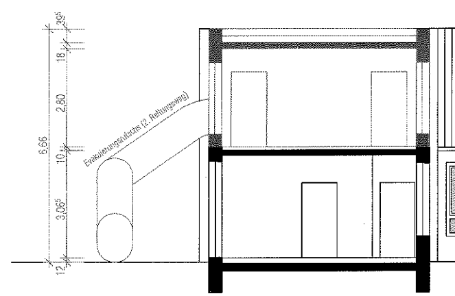
Schnitt Gruppenraum
