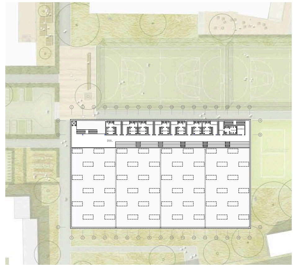
Grundriss 1. Obergeschoss
