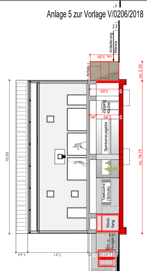
Schnitt - C-C
