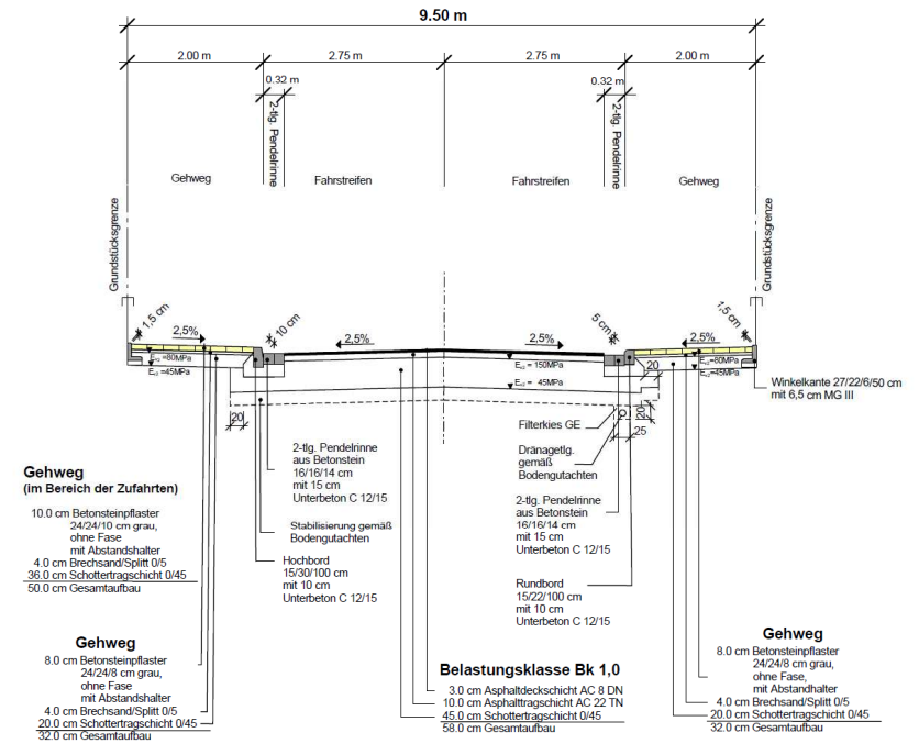
Schwarzer Kamp ( Tempo 30 ) Schnitt B-B
