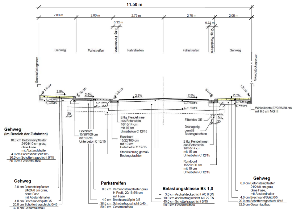
Schwarzer Kamp ( Tempo 30 ) Schnitt A-A
