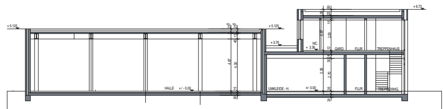
SCHNITT A-A
