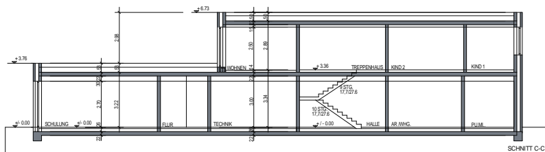
SCHNITT C-C
