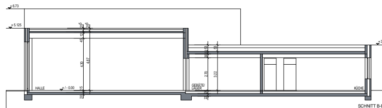
SCHNITT B-B
