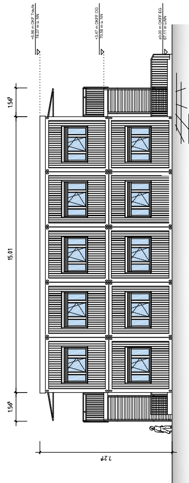
SUDANSICHT
