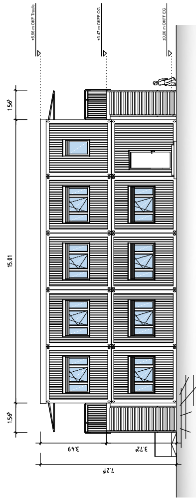
NORDANSICHT
