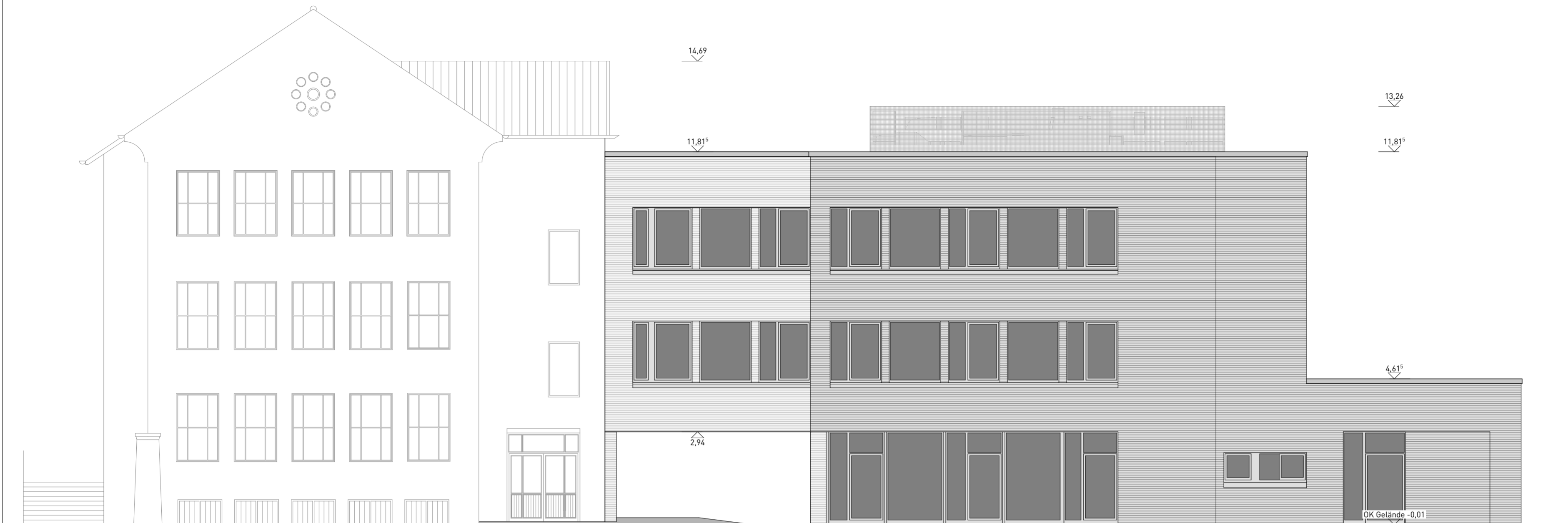
Ansicht Nord
