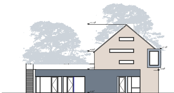
ANSICHT OSTEN
