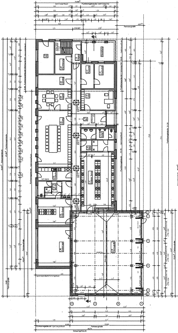
B_0_Grundriss_Erd_Obergeschoss
