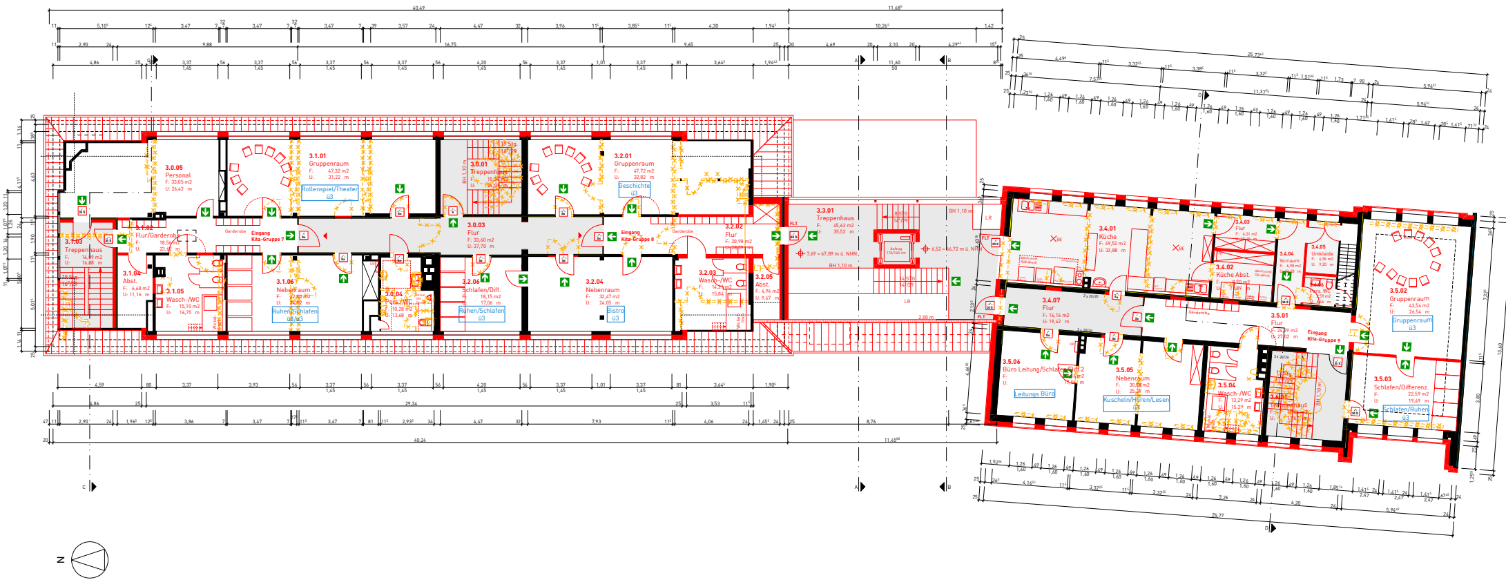
KEH_Umbau ehemaliges Hauptzollamt zu einer 9 Gruppen KiTa und 2 Großtagespflegestellen - Münster
