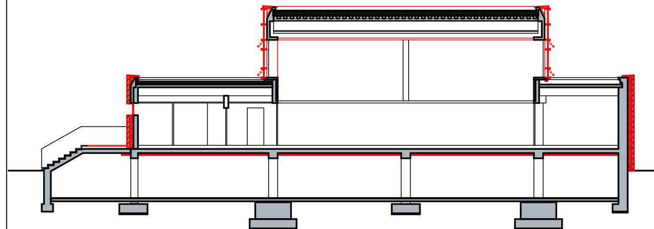
SCHNITT A-A
