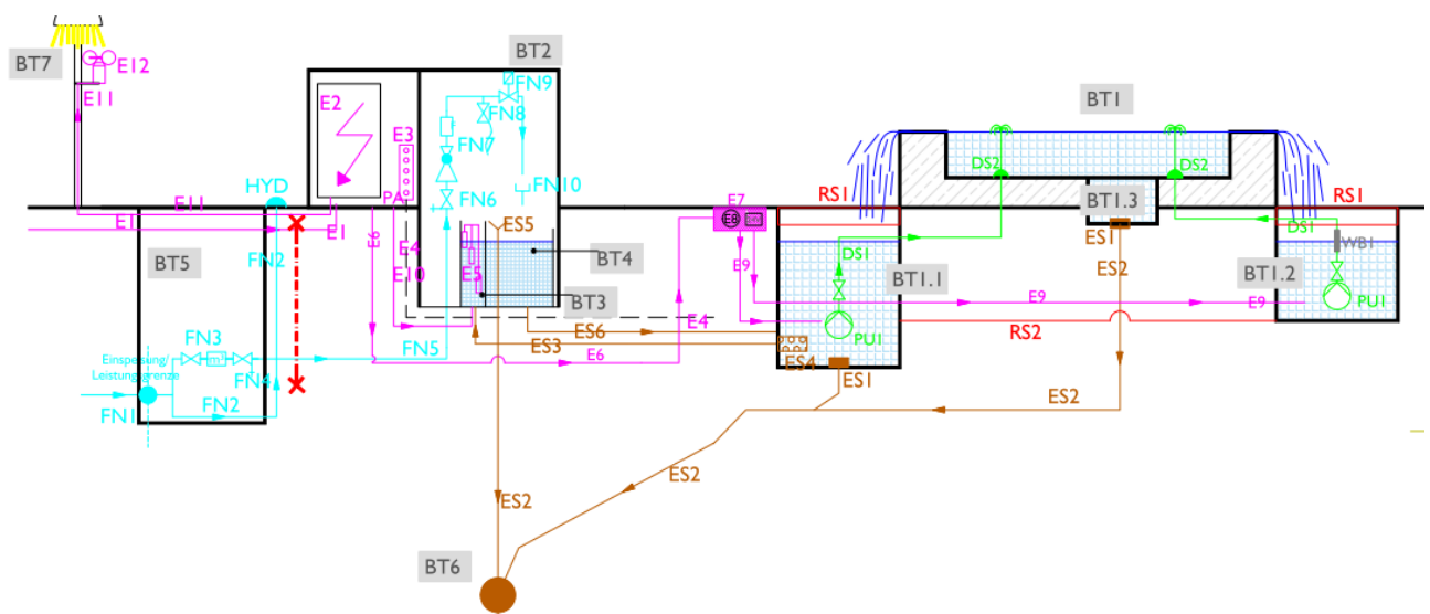
Abb. 2 Strangschema Regelsystem oberirdischen wartungsfreundlichen Niedersvoltsystem (ONS)
