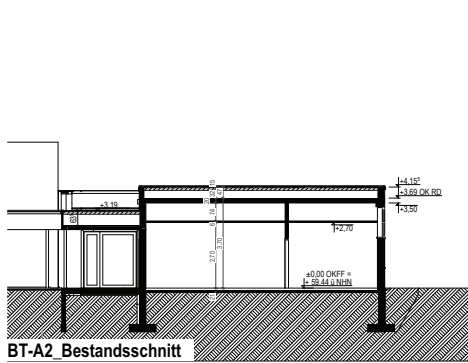
BT-A2 Bestandsschnitt
