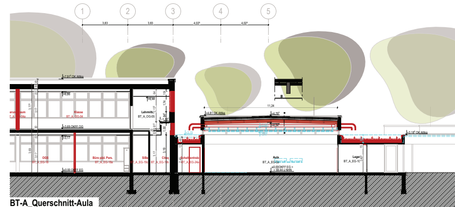
BT-A_Querschnitt-Aula
