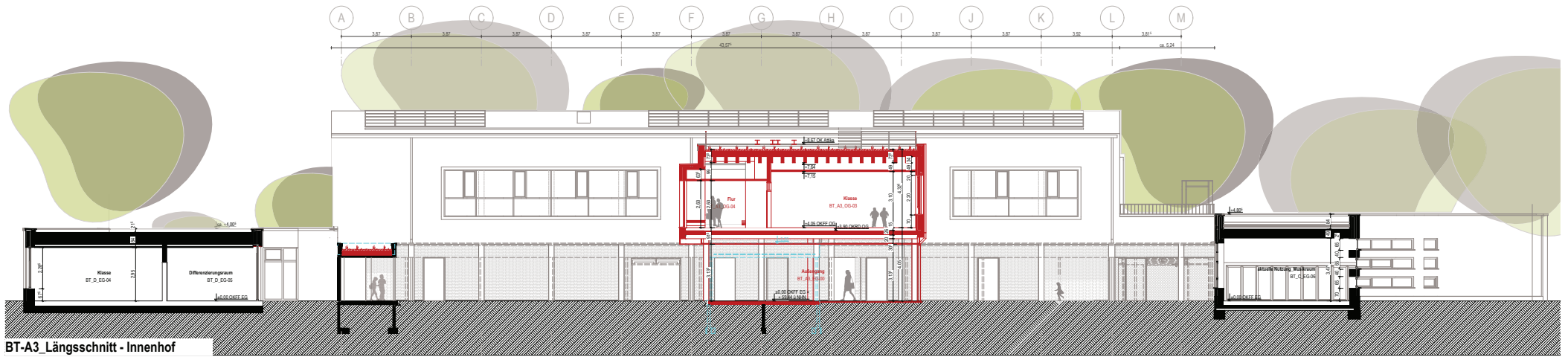
BT-A3_Längsschnitt - Innenhof
