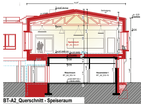
BT-A2 Querschnitt - Speiseraum
