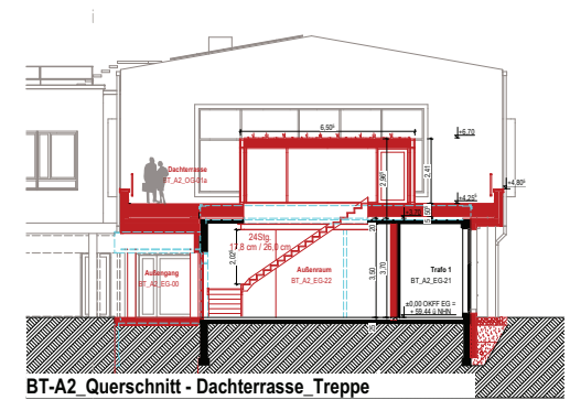
BT-A2 Querschnitt - Dachterrasse_Treppe
