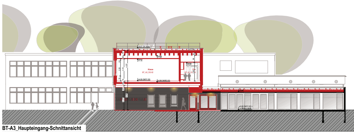
BT-A3_Haupteingang-Schnittansicht
