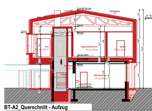
BT-A2 Querschnitt - Aufzug
