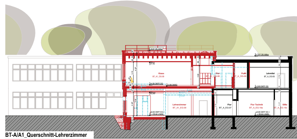
BT-A/A1_Querschnitt-Lehrerzimmer
