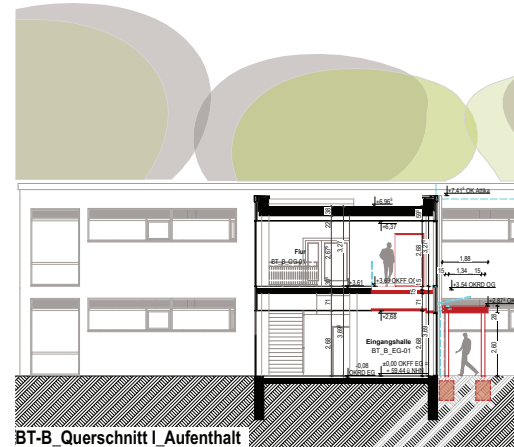
BT-B_Querschnitt I_Aufenthalt
