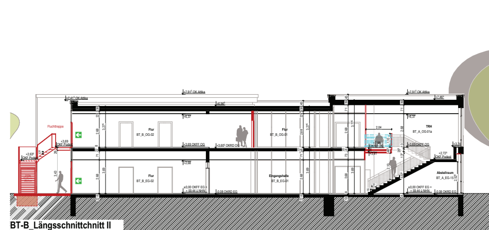
BT-B_Längsschnitt II
