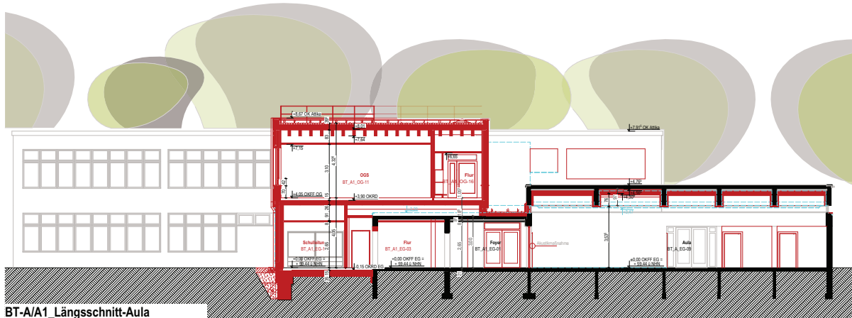
BT-A/A1_Längsschnitt-Aula
