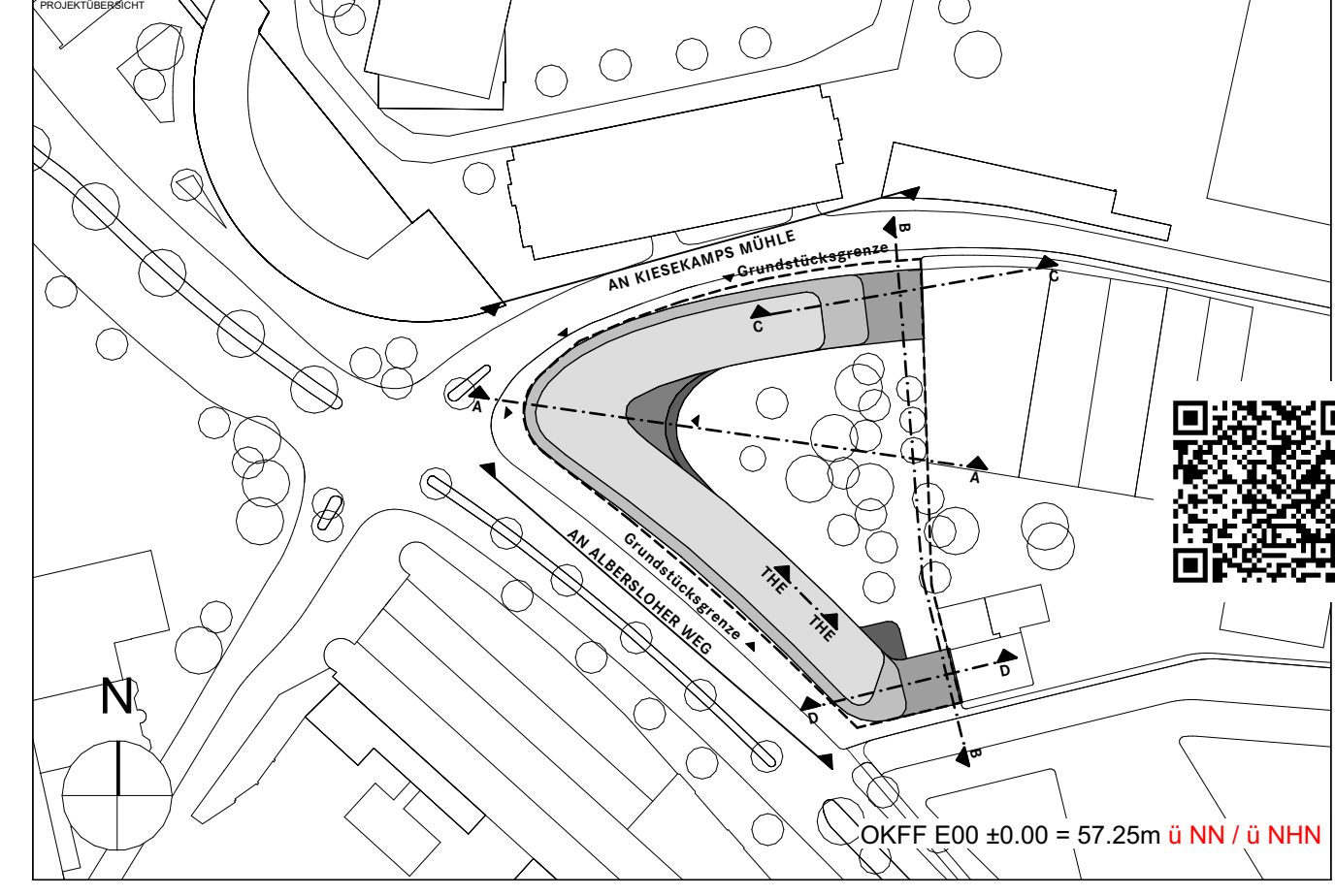
Grundriss 4. Obergeschoss 706_3_GR_04_000_05
