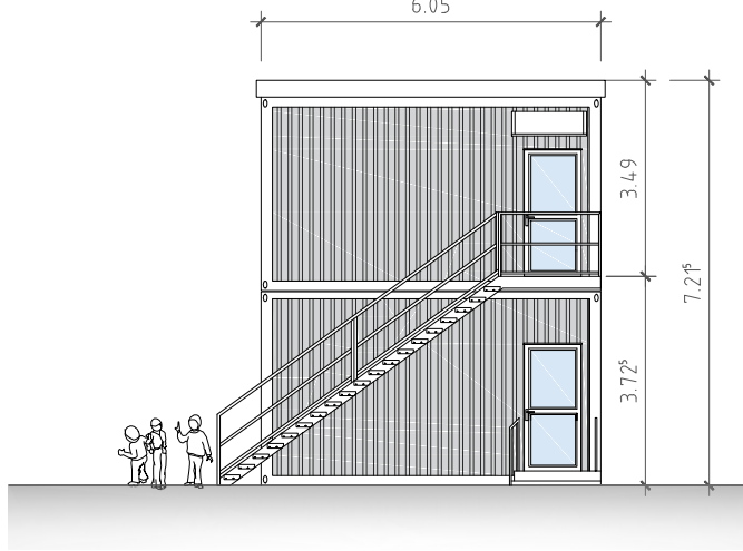
SÜDANSICHT
