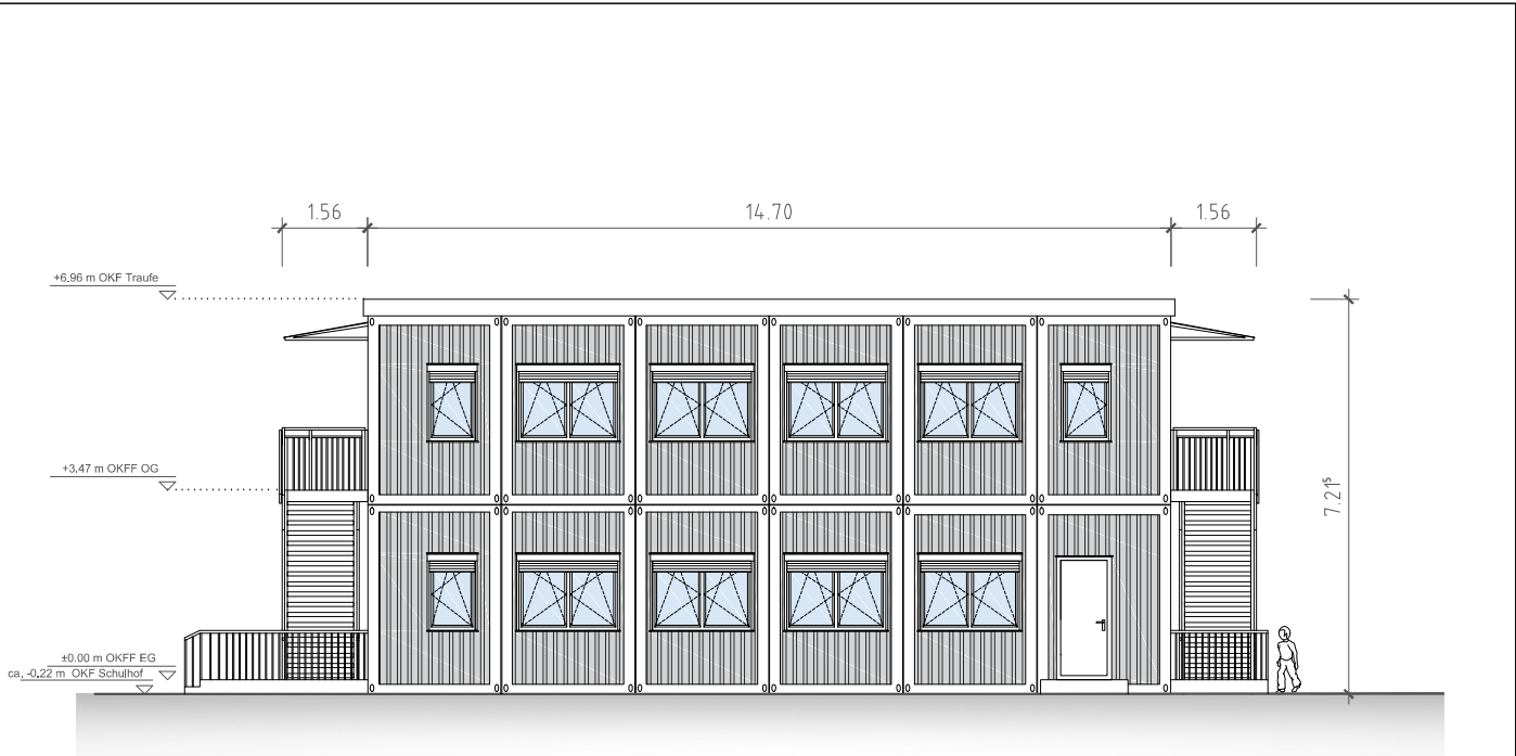
WESTANSICHT
