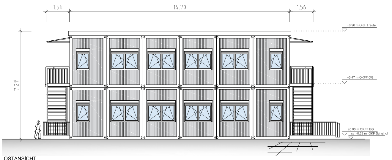
OSTANSICHT
