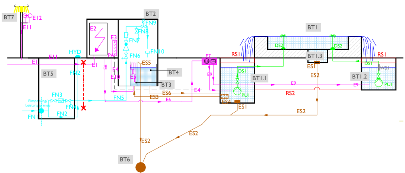
Abb. 3 Strangschema Regelsystem oberirdischen wartungsfreundlichen Niedersvoltsystem (ONS)
