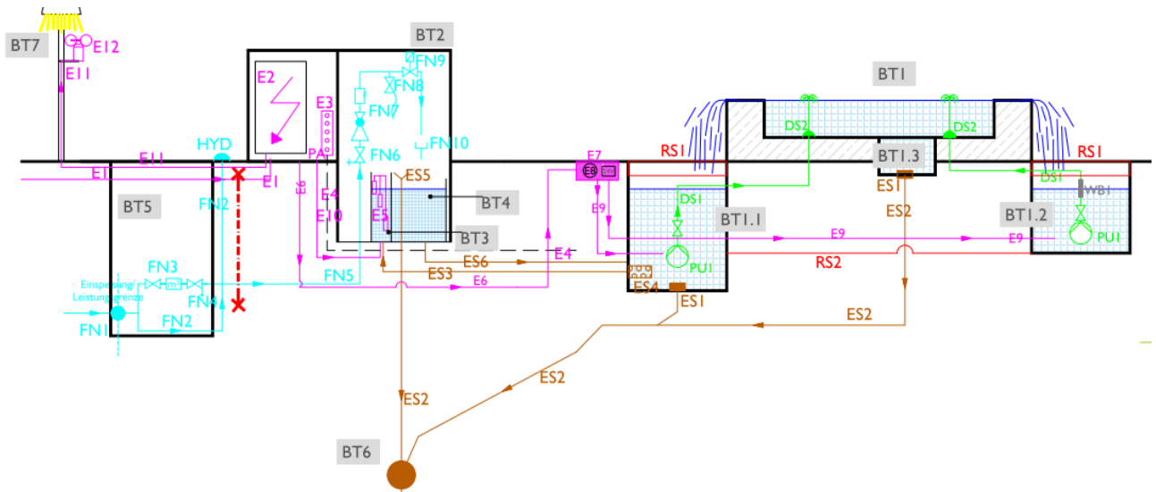
Abb. 4 Strangschema Regelsystem oberirdischen wartungsfreundlichen Niederspannungssystem (ONS)
