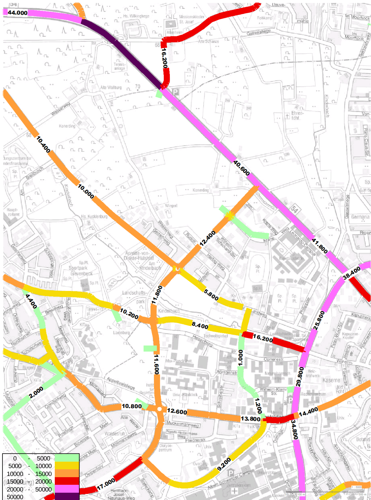
Abbildung 7 Verkehrsaufkommen im Prognoseplanfall 1 [Kfz/24h] [Kartengrundlage: Stadt Münster]
