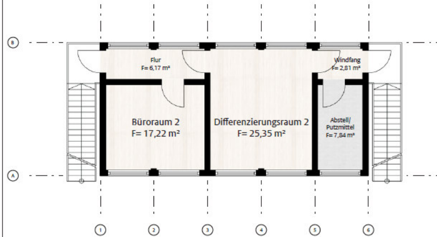
Grundriss Obergeschoss - zweigeschossig
