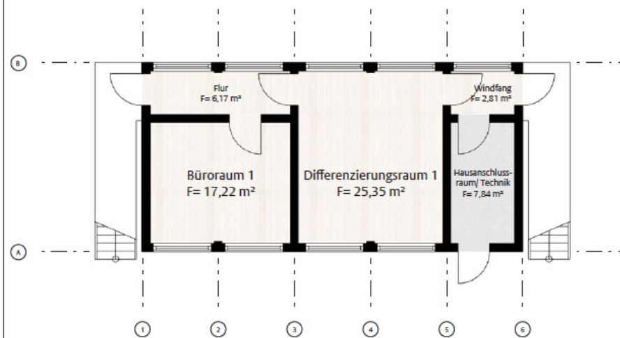
Grundriss Erdgeschoss - zweigeschossig
