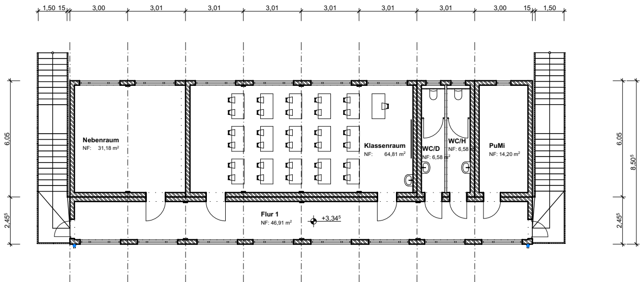
1. OBERGESCHOSS
