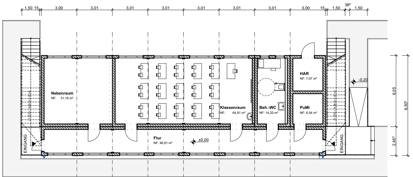
ERDGESCHOSS
