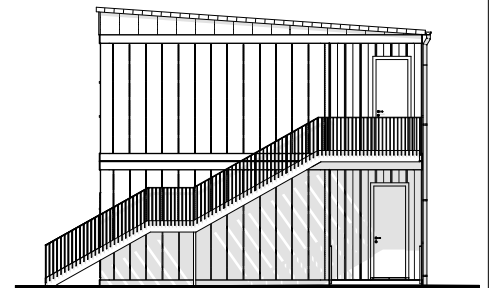
Ansicht Süd
