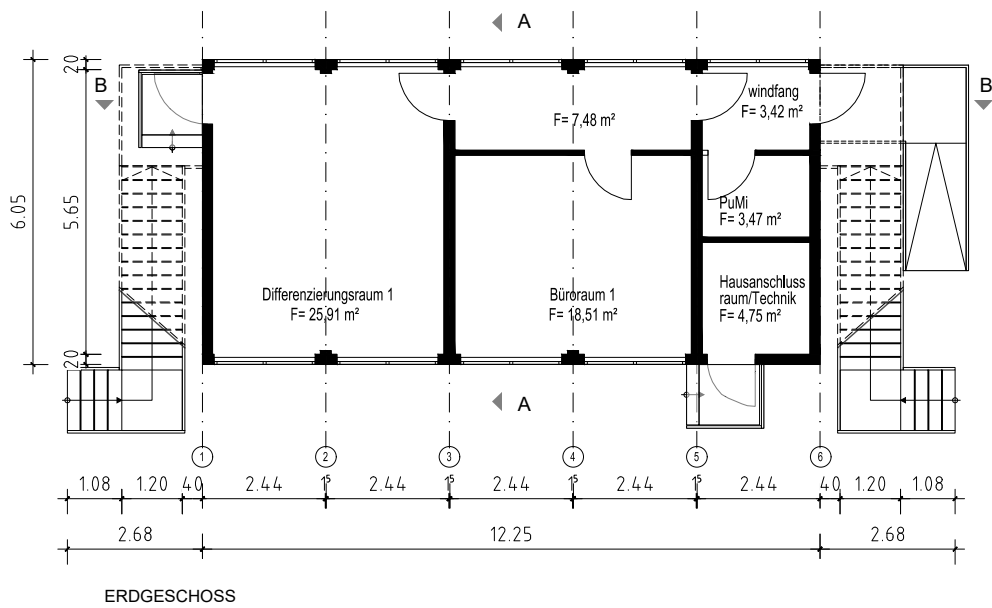
ERDGESCHOSS
