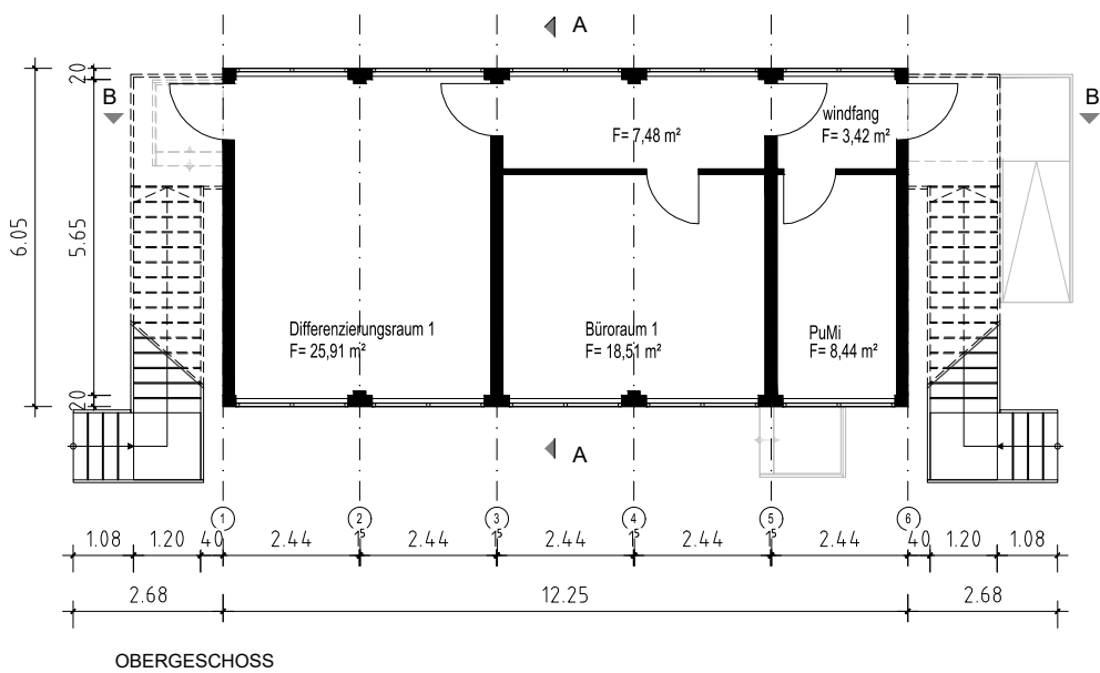
OBERGESCHOSS
