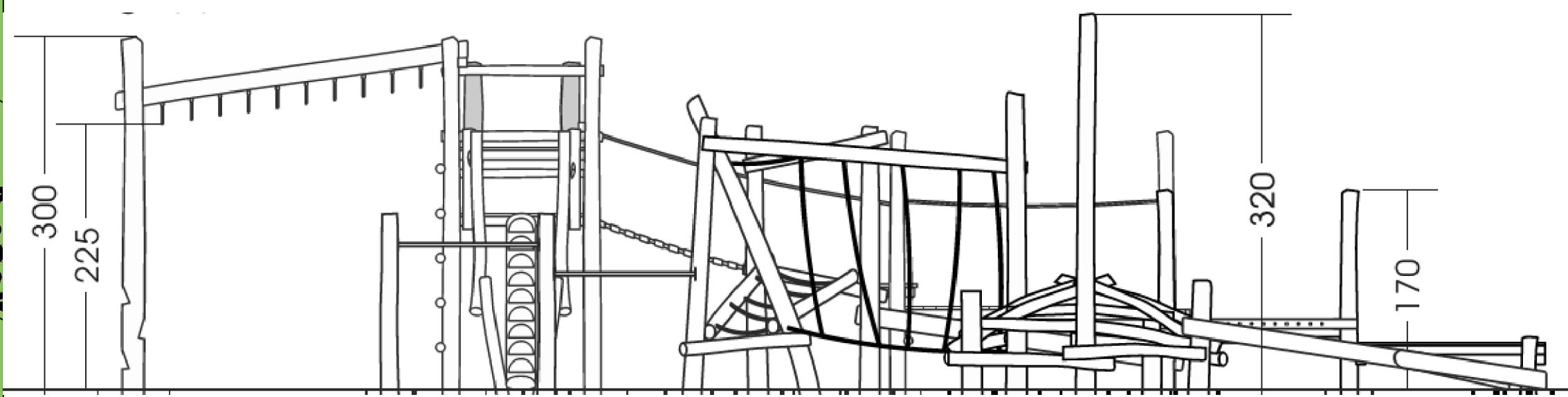
Kletterdschungel mit Hangleiter, Rutsche, Balancierelementen, Nest, Liegenetz und Umlenkpodest
