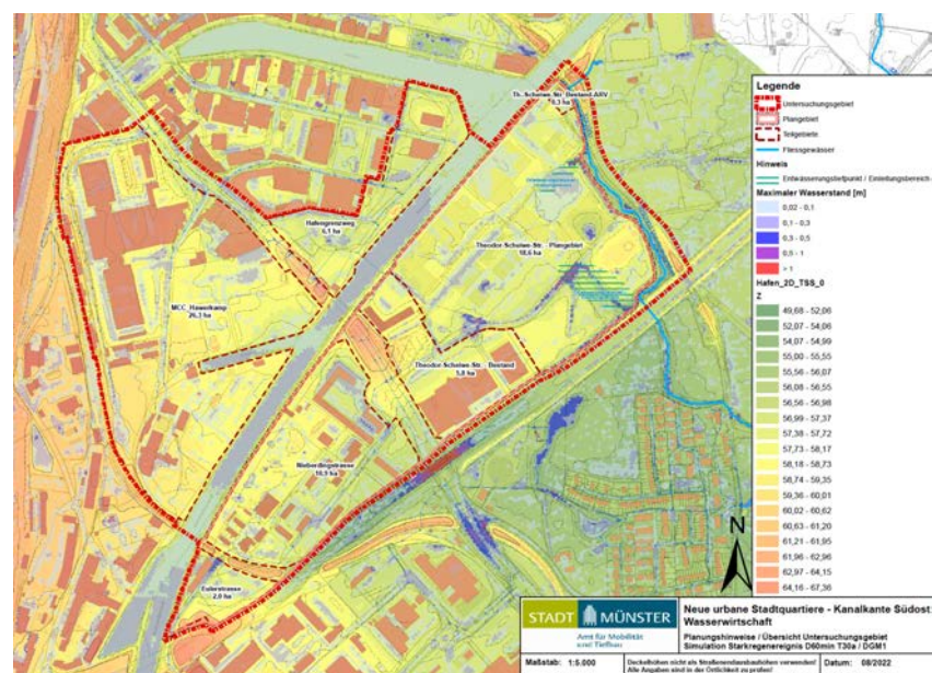
Simulation von Starkregenereignissen Areale am DEK
