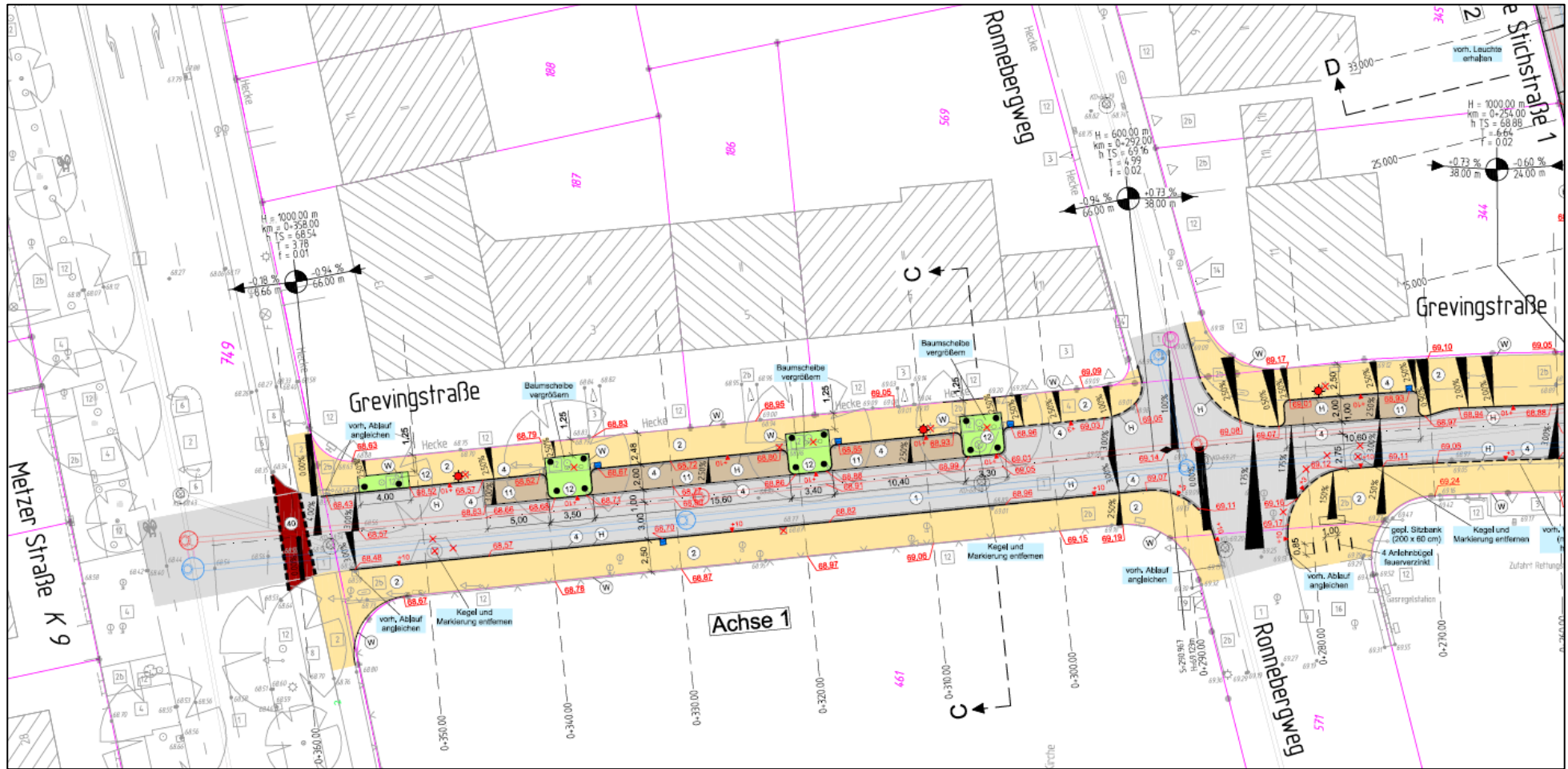
Anlage 2: Lageplan 1 (4)
