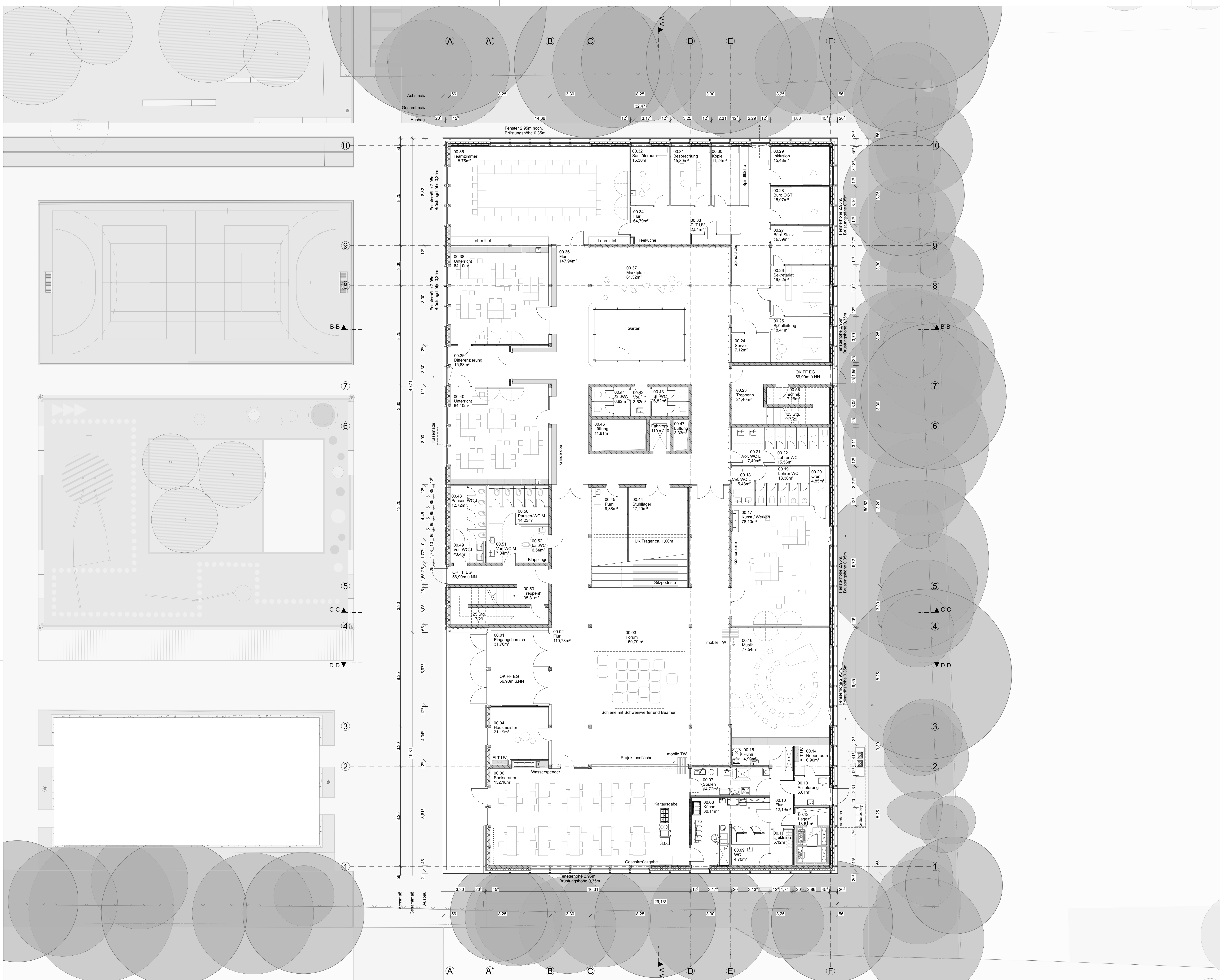
706_3_SG_GR_00_000_03_Grundriss EG
