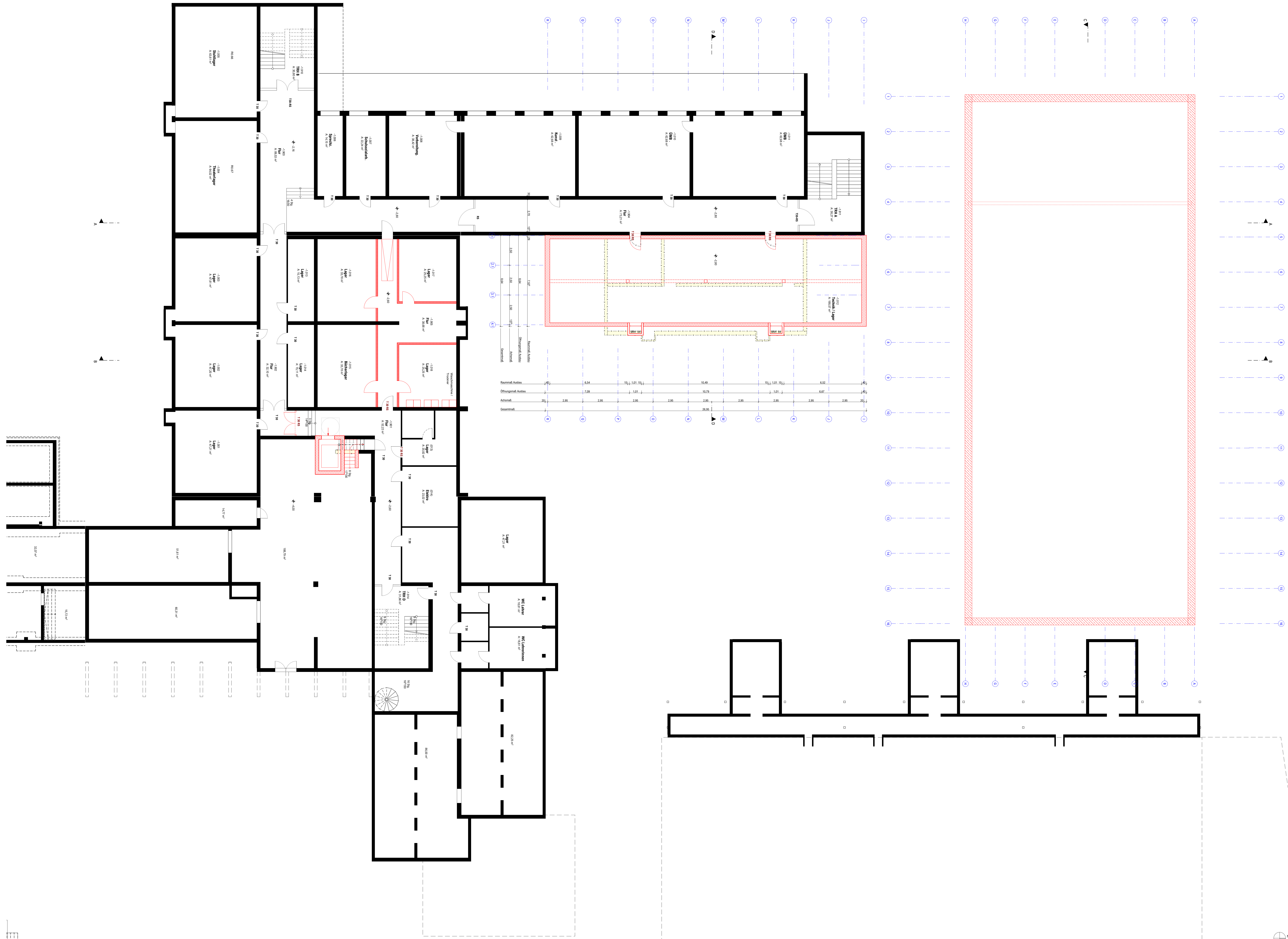
706_3_SG_GR_-1_000_02 Grundriss UG ±0,00 = 55,095 m ü.NHN
