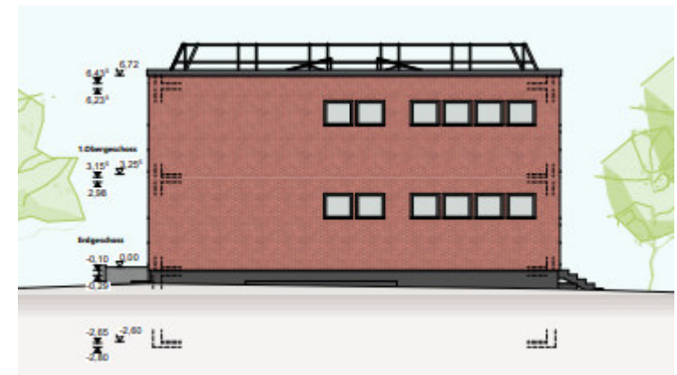
Ansicht Nord
