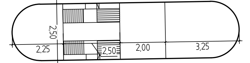
Abmessungen Querungsstelle
